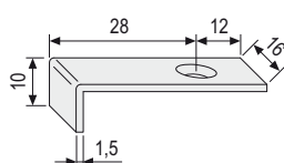
- Art. A40906.00.01 DSS, Dispositivo di sicurezza e sollevamento
