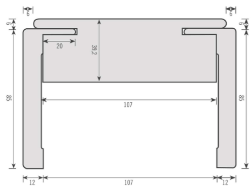
Particolare PASSATA e con ingresso "A"
