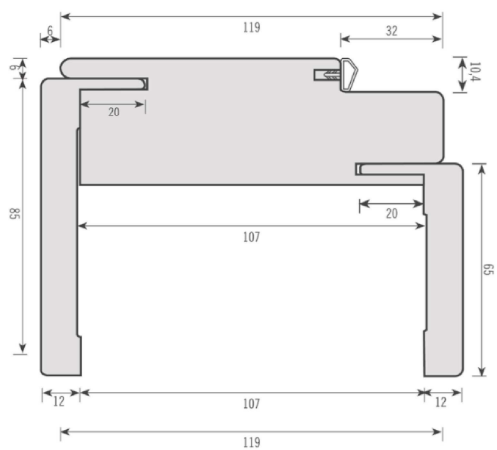
Particolare TELAIO
