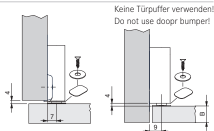
Gegenplatte zum Kleben oder Schrauben Counter part to glue or to screw
